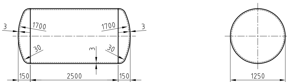
Pejletabel for 3000 liter cylindrisk liggende KN-tank
